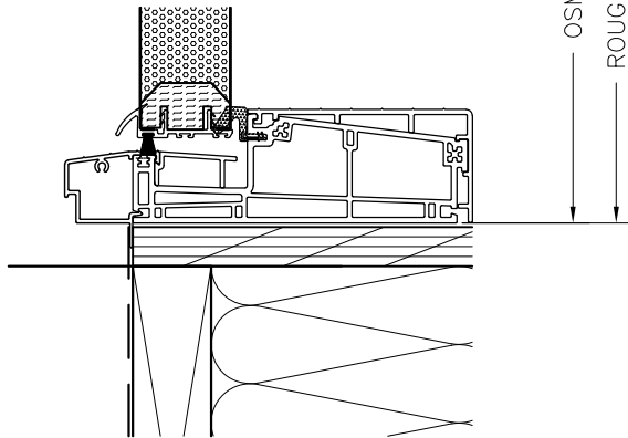
SILL DETAIL 2x6 STUD WALL
