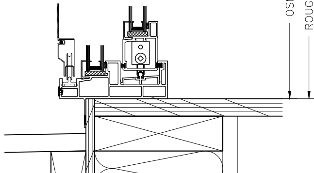
SILL DETAIL 2x6 STUD WALL
