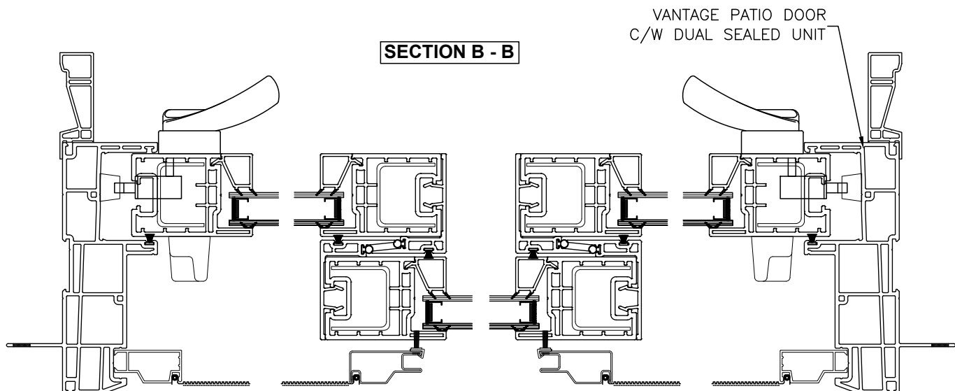
JAMB DETAIL FRAME DIMENSIONS
