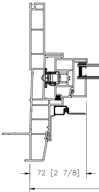
JAMB DETAIL FRAME DIMENSIONS
