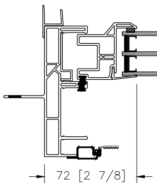
JAMB DETAIL FRAME DIMENSIONS
