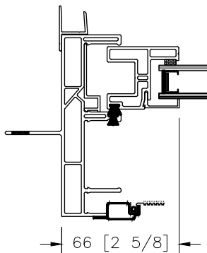
JAMB DETAIL FRAME DIMENSIONS
