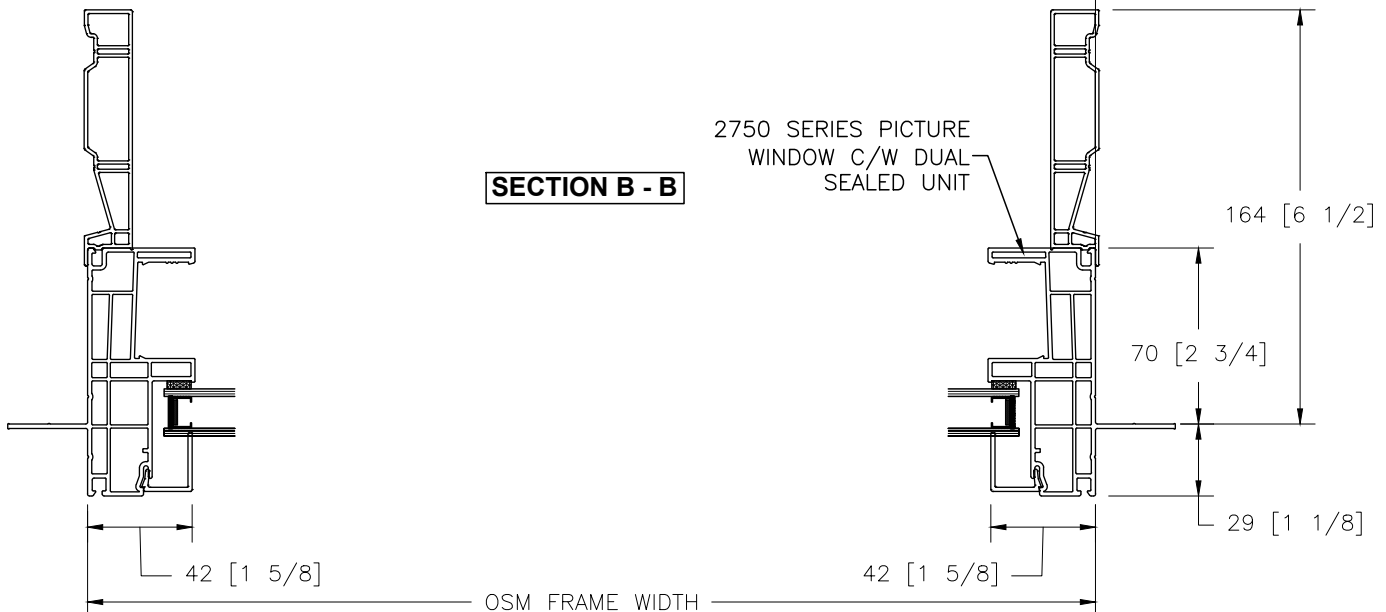
JAMB DETAIL FRAME DIMENSIONS
