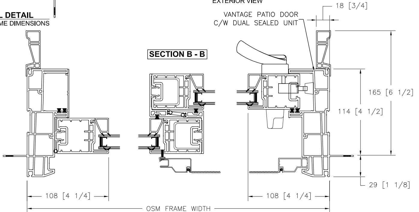
JAMB DETAIL FRAME DIMENSIONS
