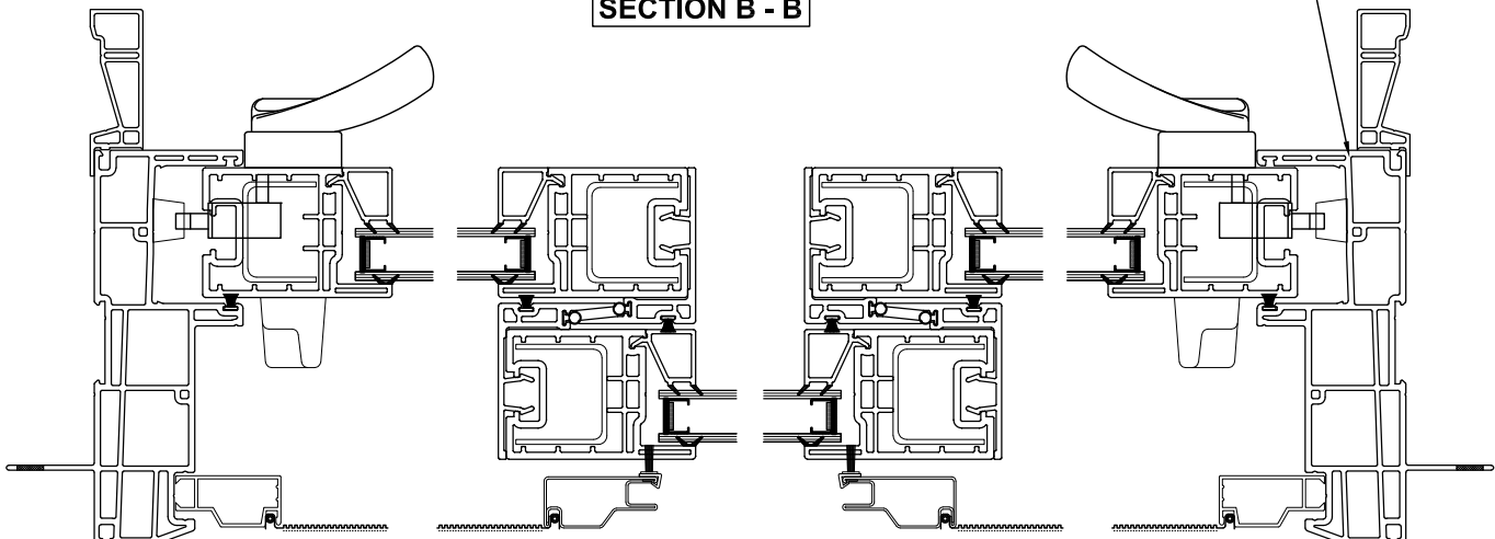
JAMB DETAIL FRAME DIMENSIONS
