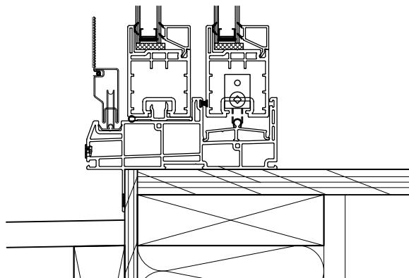
SILL DETAIL 2x6 STUD WALL
