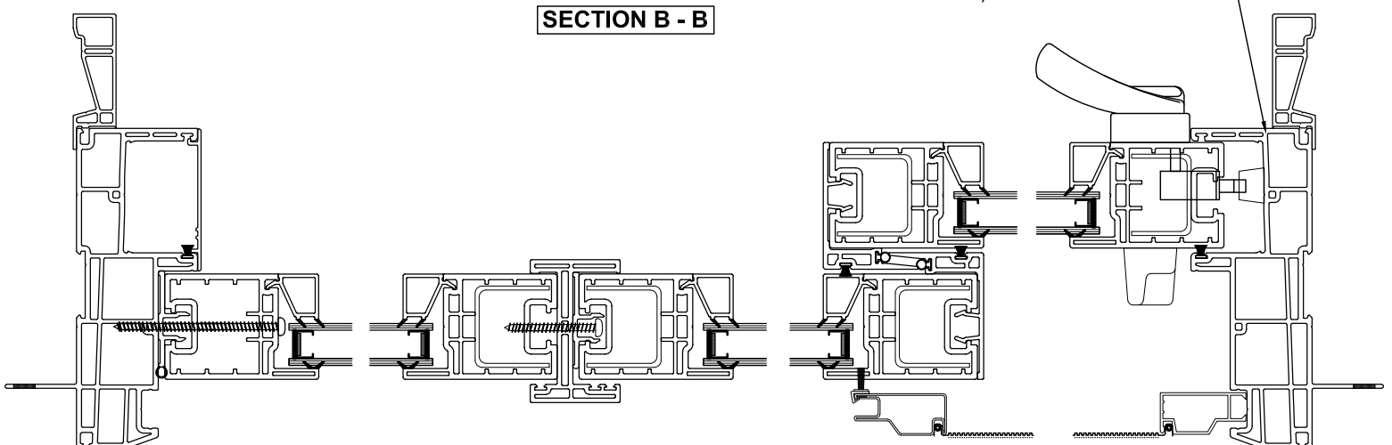
JAMB DETAIL FRAME DIMENSIONS
