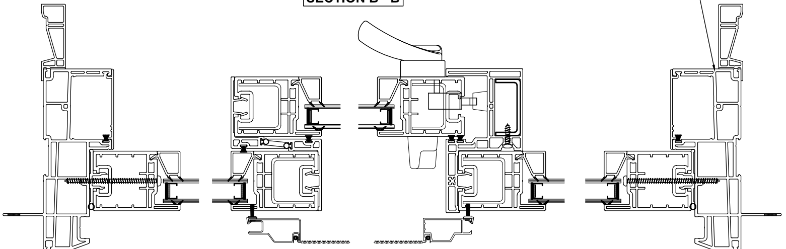
JAMB DETAIL FRAME DIMENSIONS
